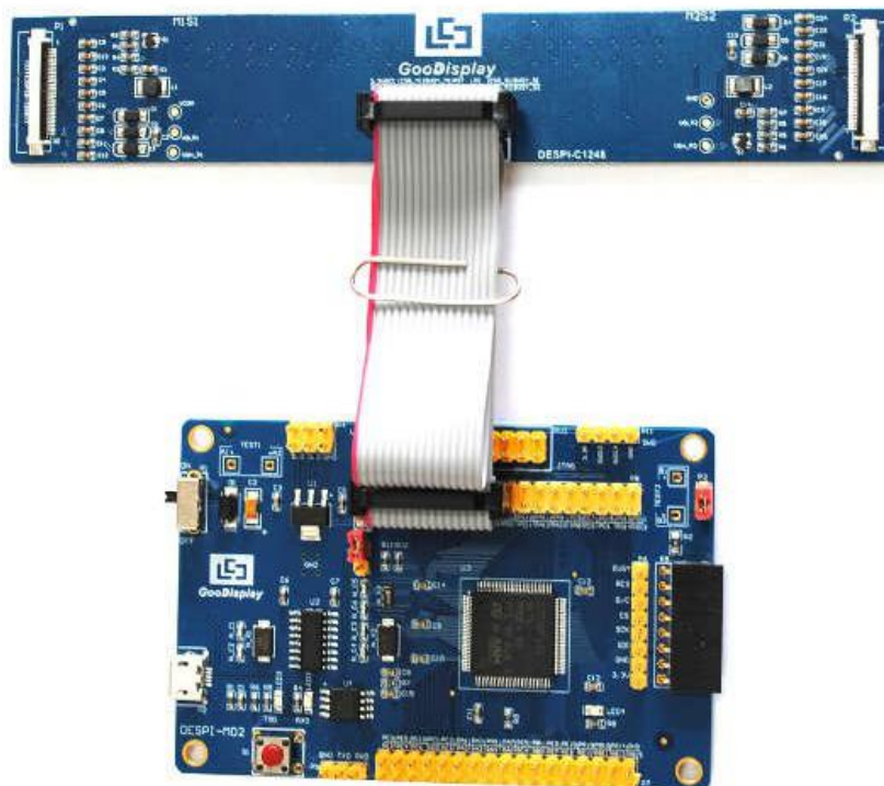
图 3 主板与转接板连接方式
