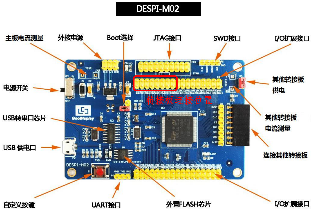
图 1 DESPI-M02 主板功能图
