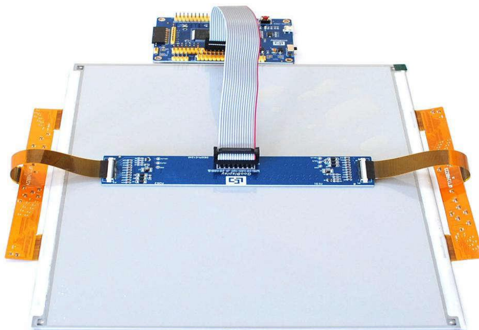
图 10 完整连接图
