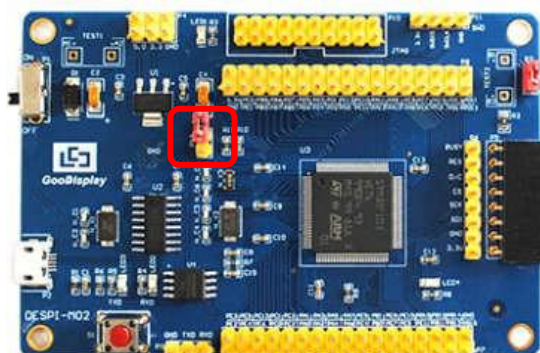
图 17 P12 短接位置
